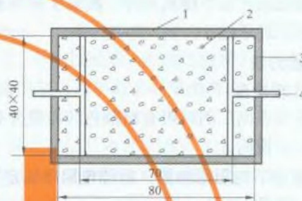
1—绝缘板；2—降阻剂； 3—绝缘盒；4—铜电极
