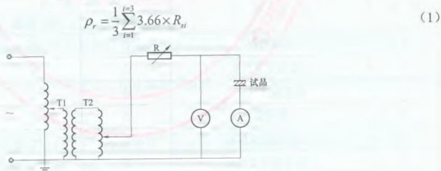
图4 试品电阻测量回路
